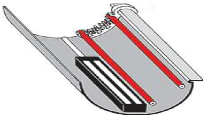
Montaż czujnika w rynnie
