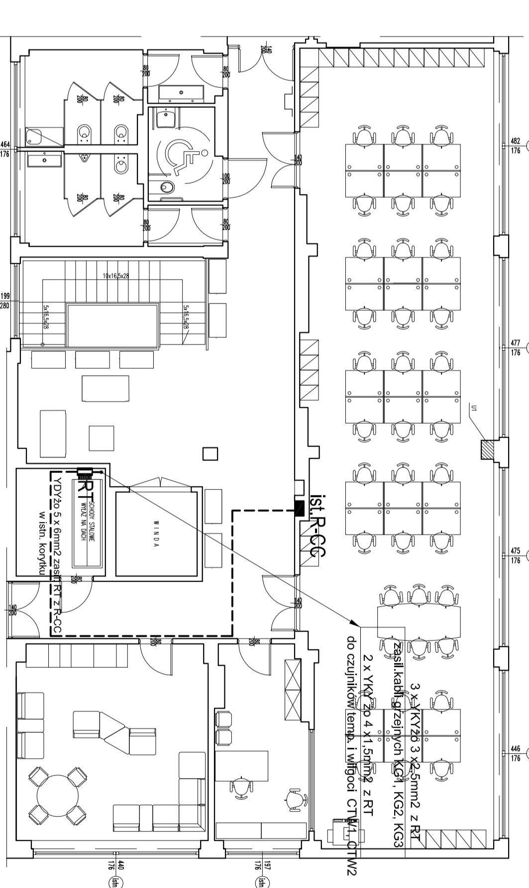
RZUT II PIĘTRA / fragment / skala 1:50
